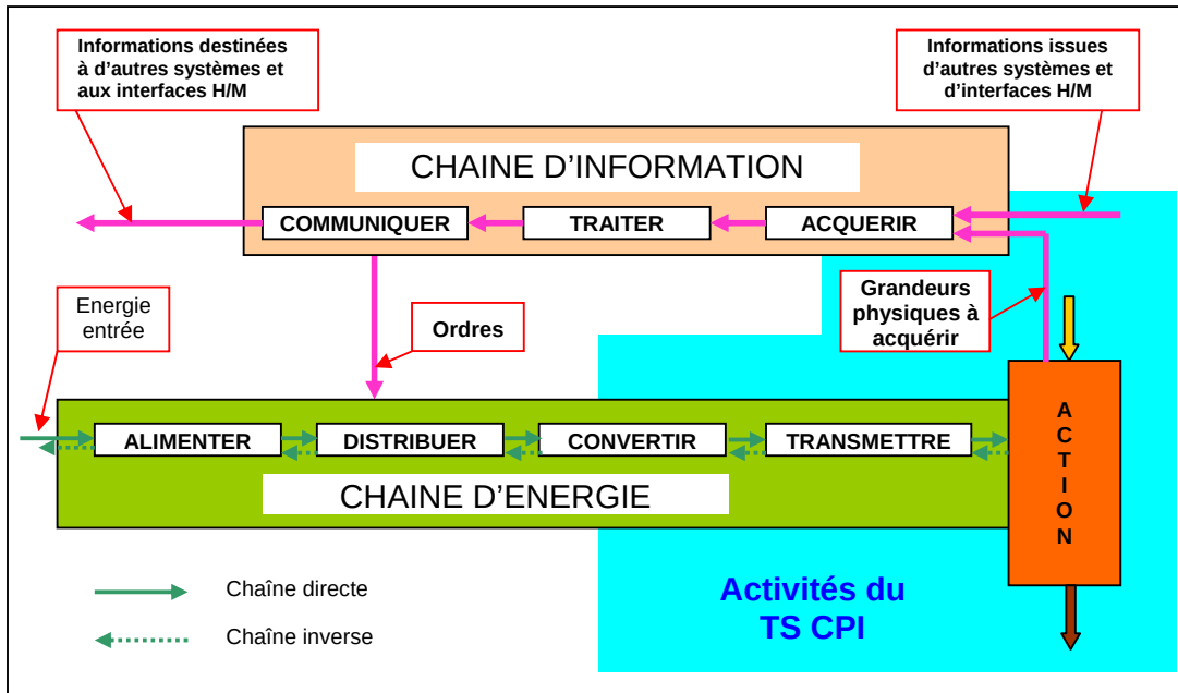
Figure 3 : architecture fonctionnelle générique des produits pluri techniques
